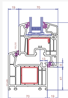
PERFIL DE 70 mm.
